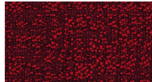
Garnet
